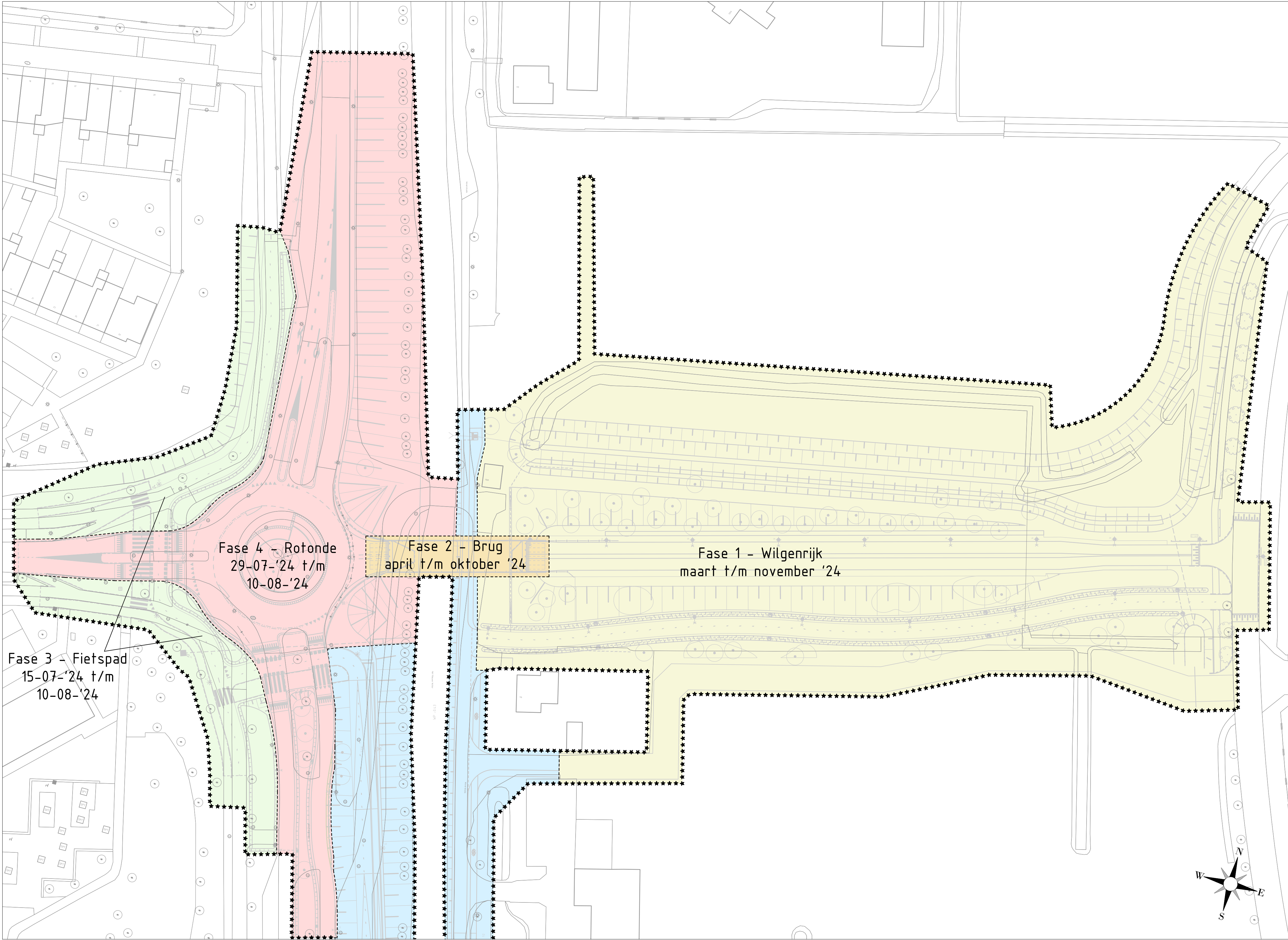
Situatie hoofdontsluiting SCHAAL 1 : 500
